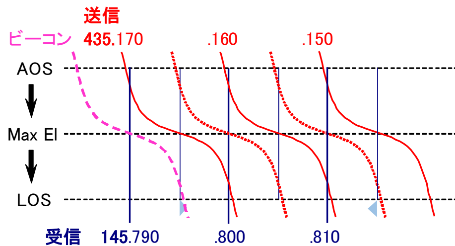
XW-2C 送信-受信周波数
