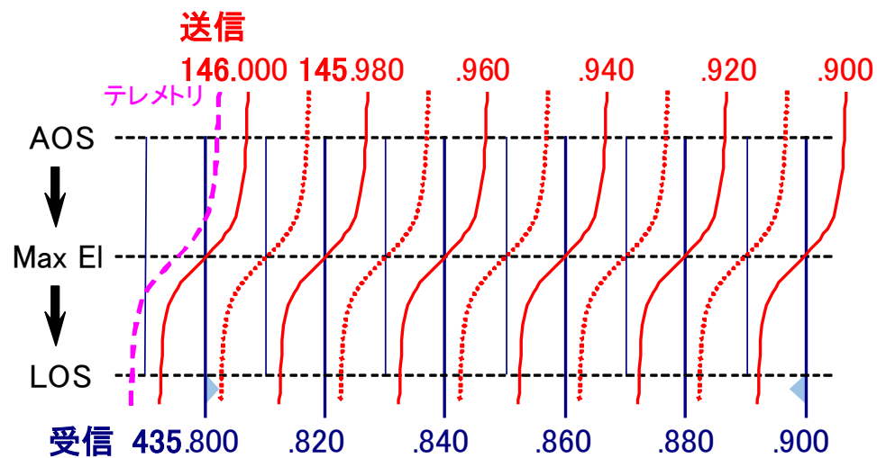
FO-29 送信-受信周波数
