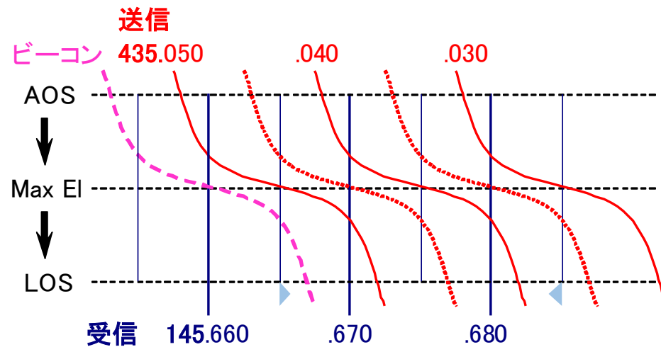
XW-2A 送信-受信周波数
