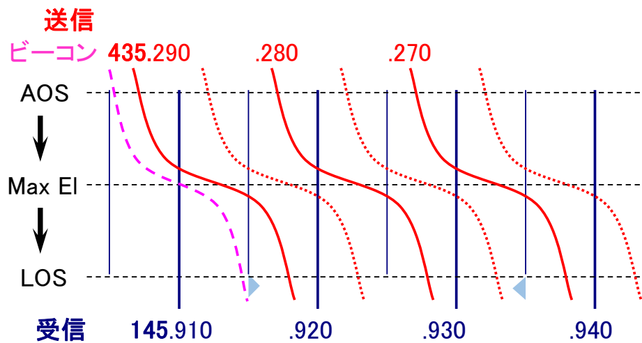
CAS-4B 送信-受信周波数
