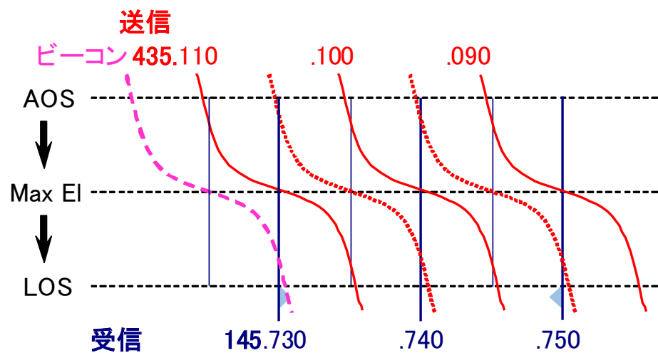
XW-2B 送信-受信周波数
