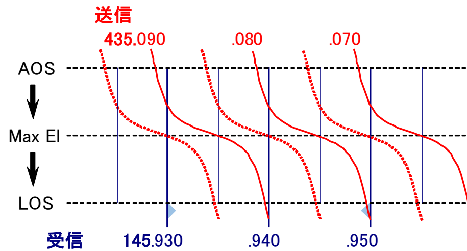
UKube-1 送信-受信周波数
