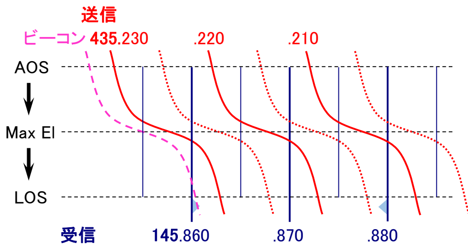
XW-2D 送信-受信周波数
