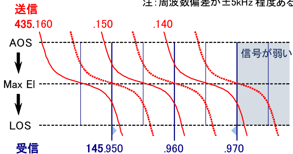
AO-73 送信-受信周波数
