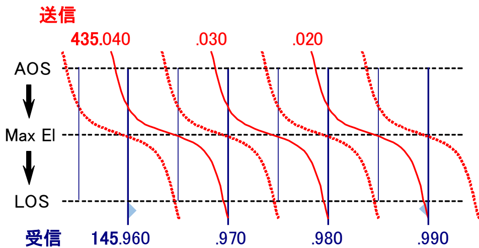
EO-88 (Nayif-1) 送信-受信周波数
