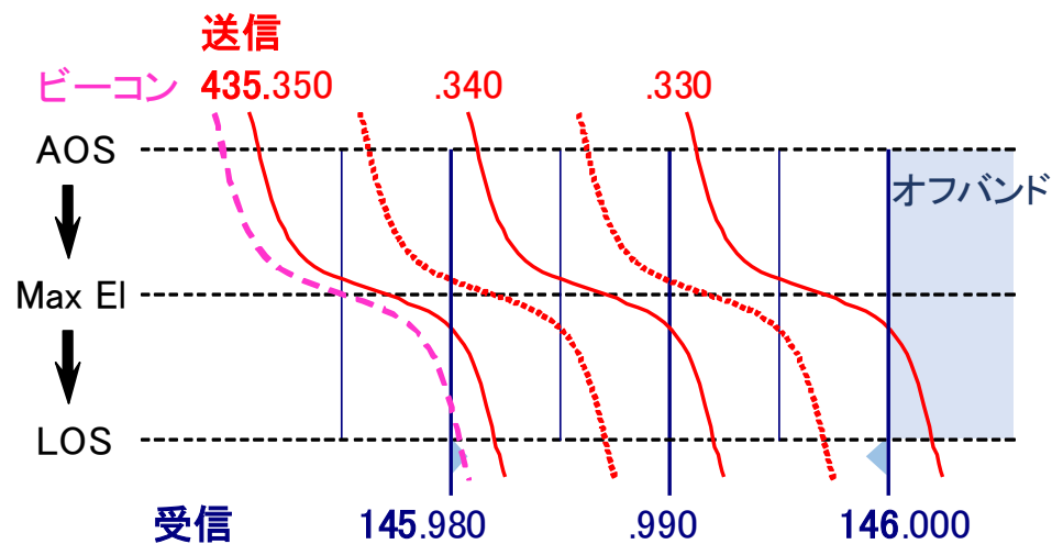
XW-2F 送信-受信周波数
