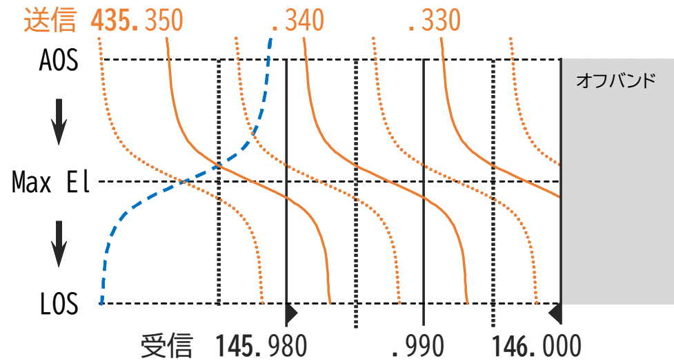
XW-2F 送信-受信周波数 by JO2ASQ
